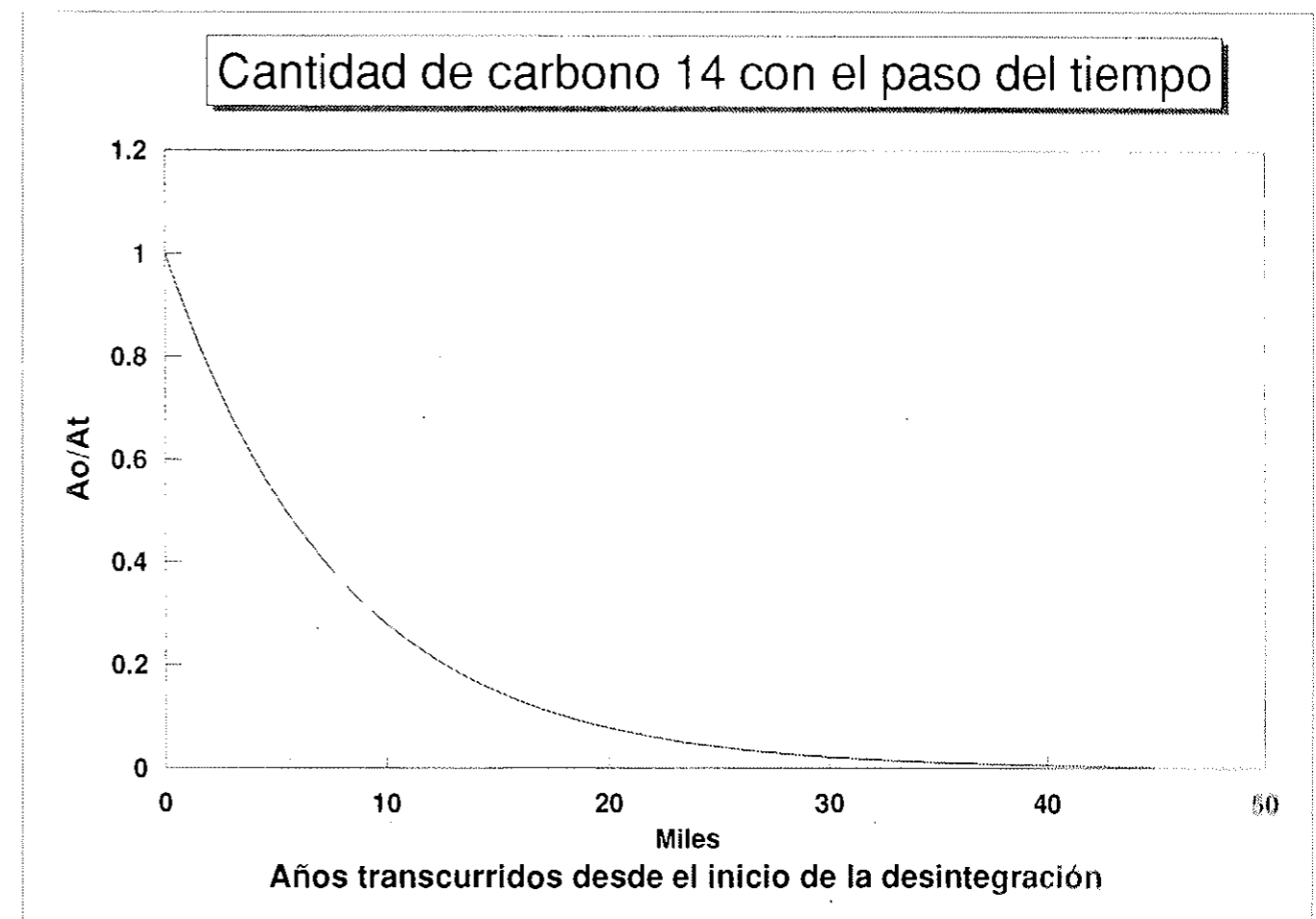
Figura 1.- Los isótopos radiactivos son aquellos elementos que se desintegran en otros. El caso más simple es el de un elemento A que se desintegre en otro elemento no radiactivo (estable) B. En la figura mostramos un ejemplo de este tipo. Corresponde al carbono-14 que se desintegra en nitrógeno-14. En otros casos el proceso es más complicado. A veces ocurre que un elemento A se desintegra en otro B, también sea radiactivo, que a su vez se desintegra en otro C. La velocidad de desintegración de un elemento se suele expresar por el período de semidesintegración, que se define como el tiempo necesario para que se desintegren la mitad de los átomos del elemento. En el caso del carbono-14 este valor es de 5.430 años. Eso significa que partiendo de una cantidad 1, pasados 5.430 años quedará 1/2 y transcurridos otros 5.430 años quedará 1/4 y así sucesivamente. Esta propiedad se utiliza para determinar la edad de rocas, objetos, etc. Naturalmente se necesita que se den condiciones para ello, como por ejemplo que el objeto contenga, en cantidad detectable, un isótopo apropiado a la edad que se pretende medir.
